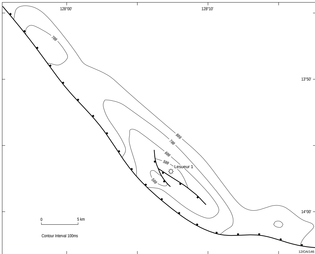
Lesueur, Top Permian, TWT map
