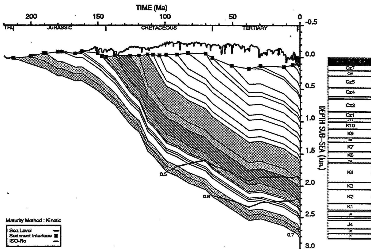
GEOHISTORY PLOT : Lombardina 1
