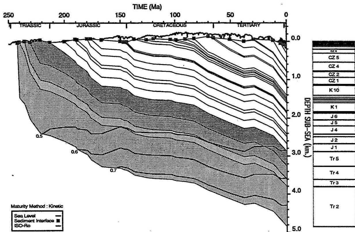
GEOHISTORY PLOT : Phoenix 1
