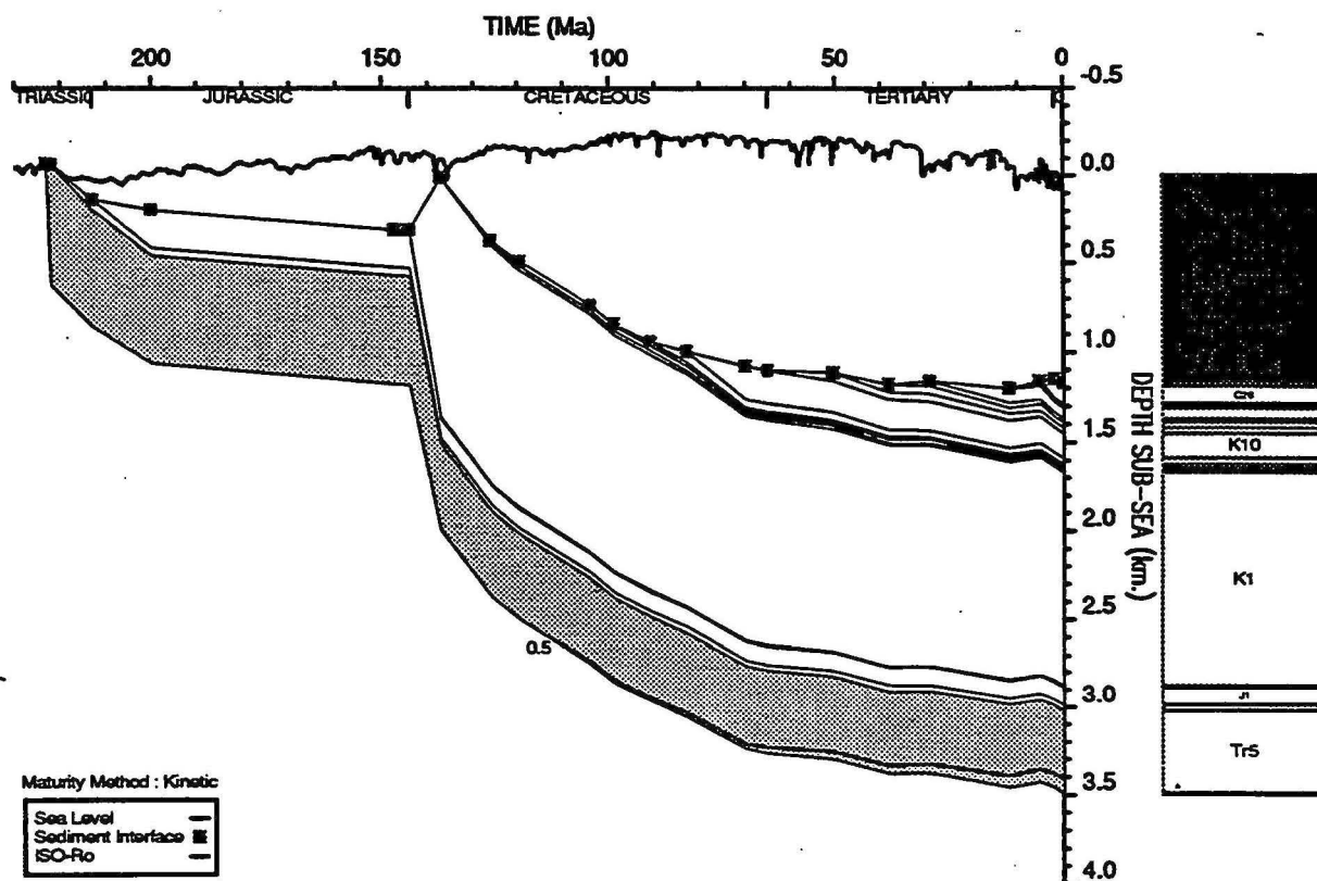
GEOHISTORY PLOT : Sirius 1
