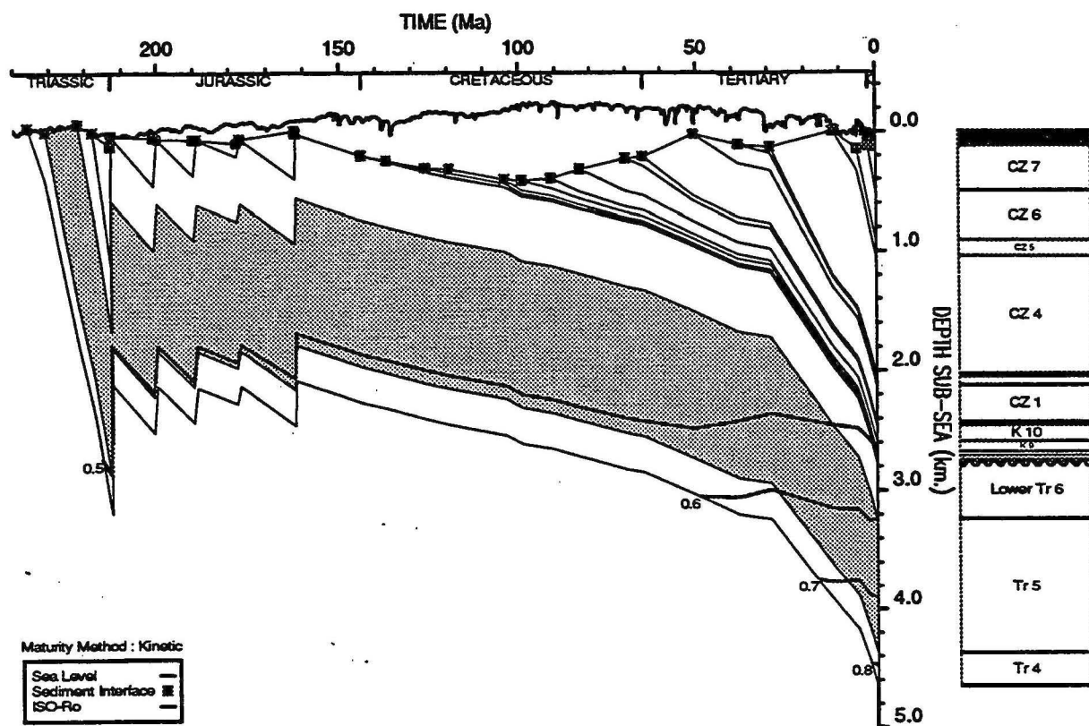
GEOHISTORY PLOT : Goodwyn 6
