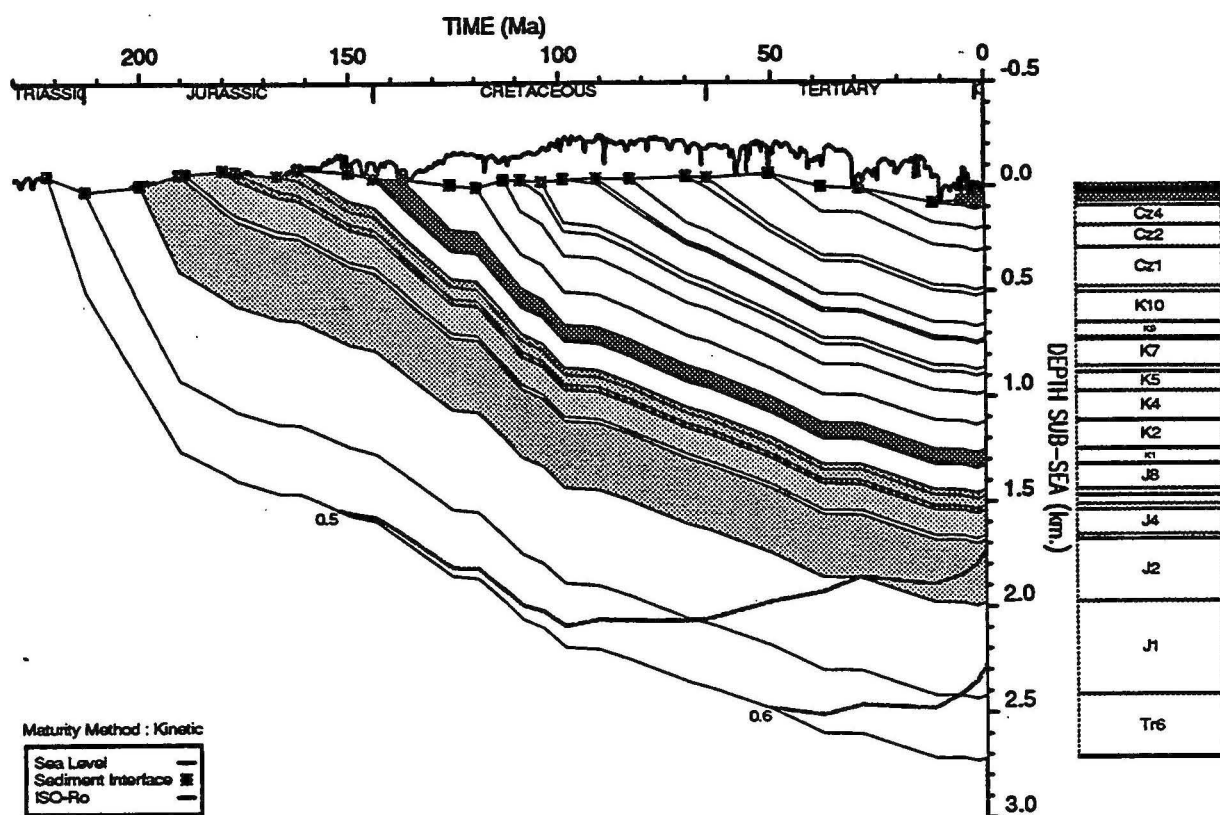
GEOHISTORY PLOT : Lynher 1
