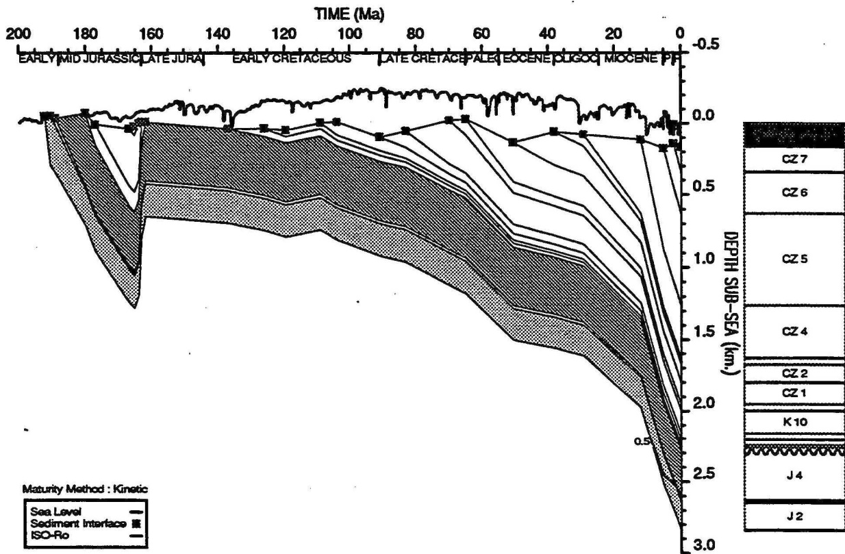
GEOHISTORY PLOT : Ronsard 1
