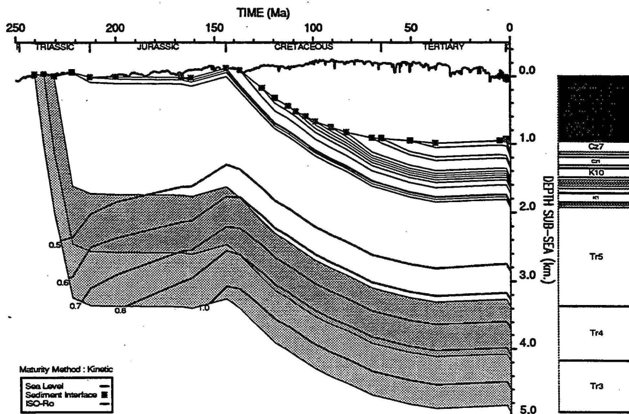
GEOHISTORY PLOT : Jupiter 1
