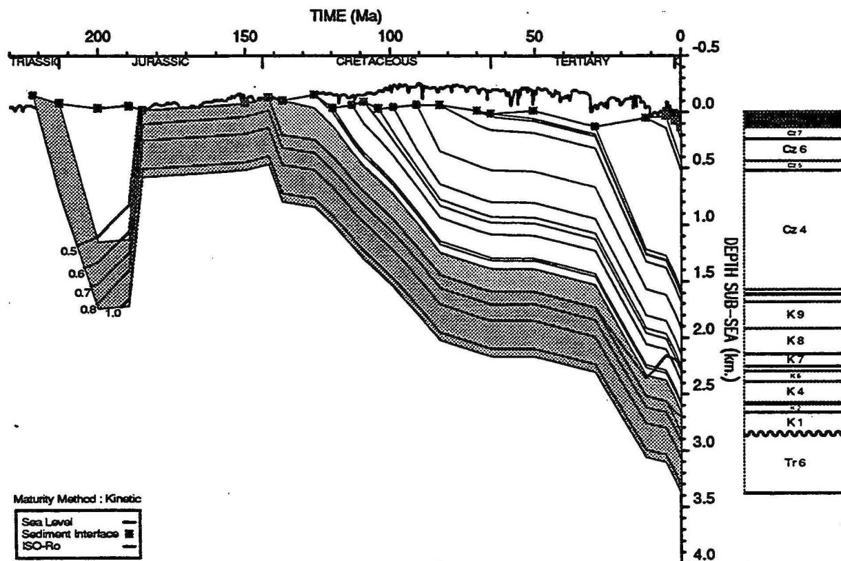
GEOHISTORY PLOT : Griffin 1
