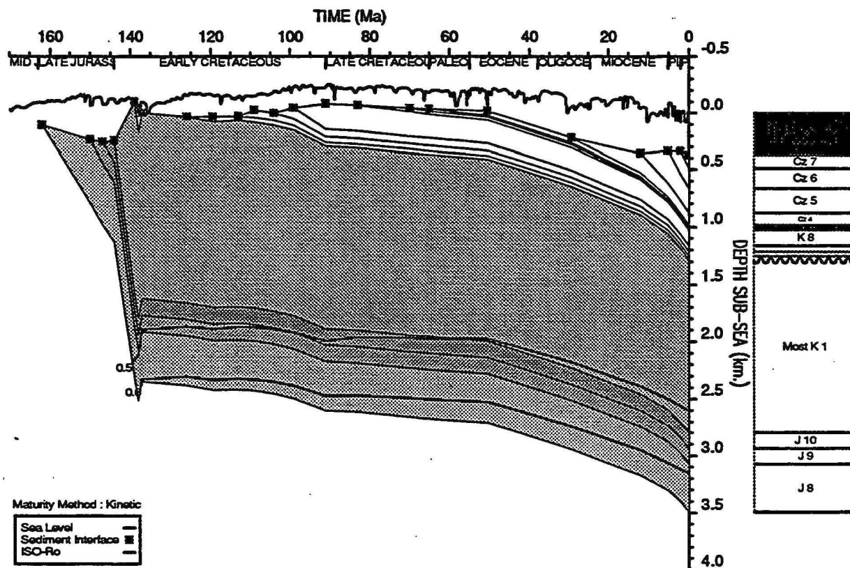
GEOHISTORY PLOT : Novara 1
