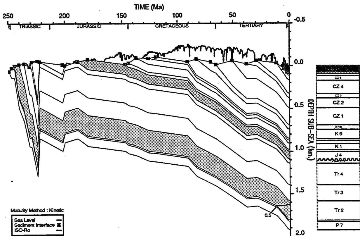
GEOHISTORY PLOT : Poissonnier 1
