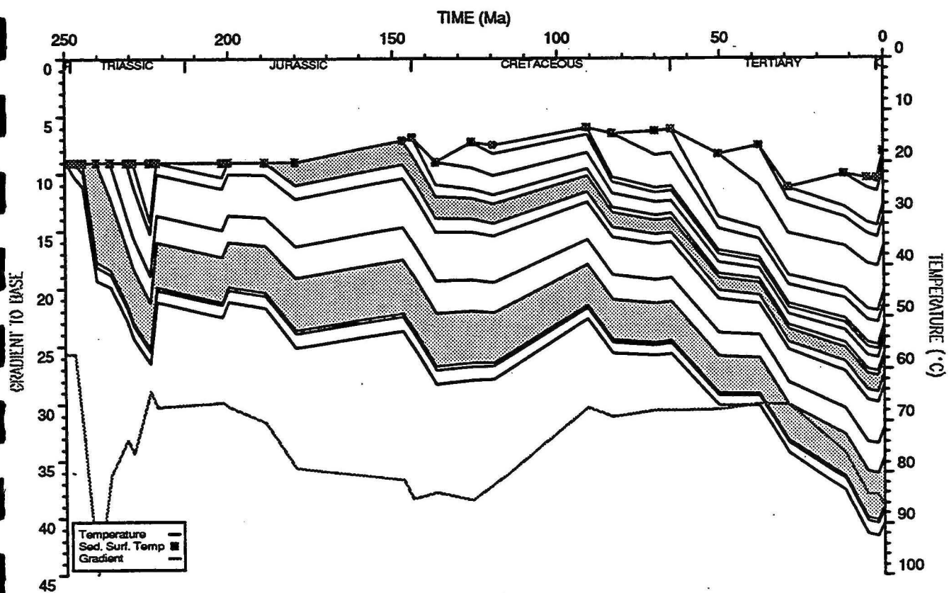
BED TEMPERATURE PLOT : Poissonnier 1
