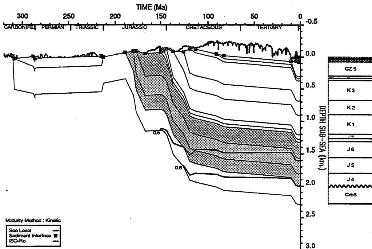
GEOHISTORY PLOT : Lapeche 1A
