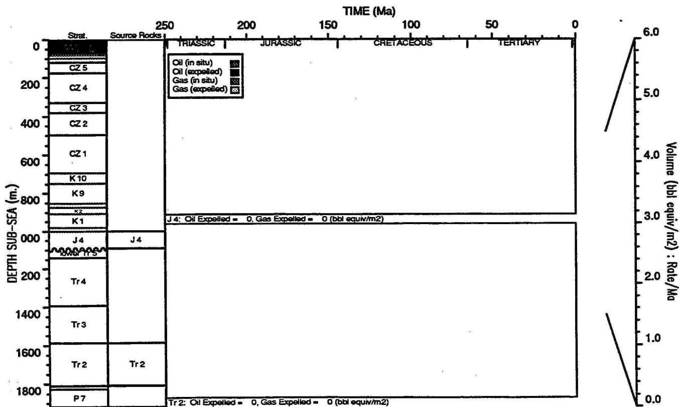
HYDROCARBON GENERATION PLOT : Poissonnier 1
