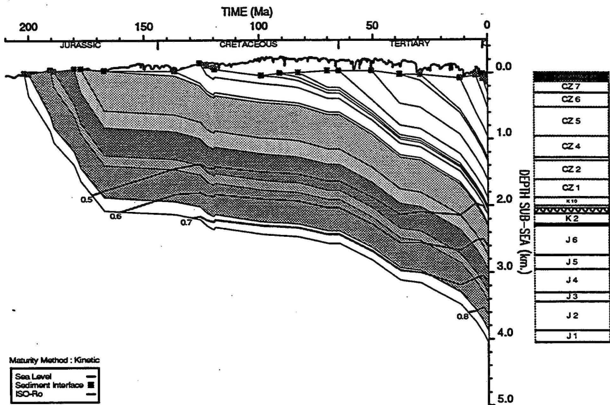
GEOHISTORY PLOT : Picard 1
