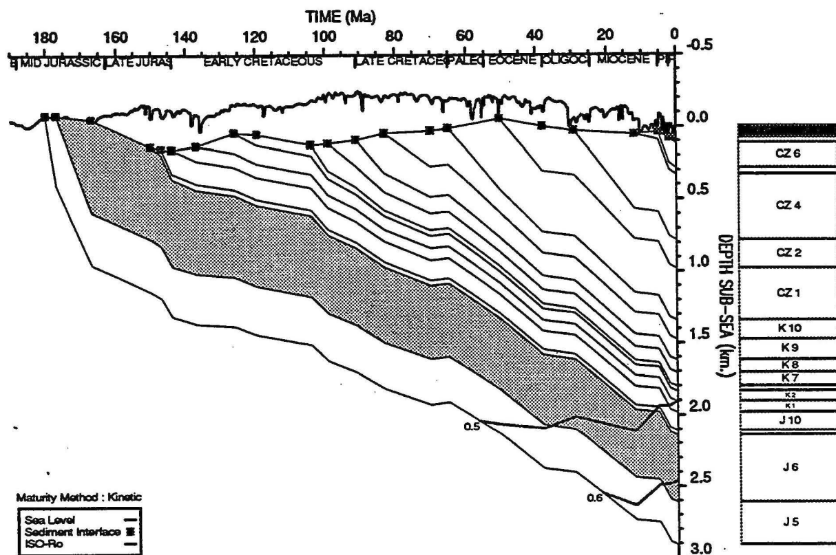
GEOHISTORY PLOT : Talisman 1
