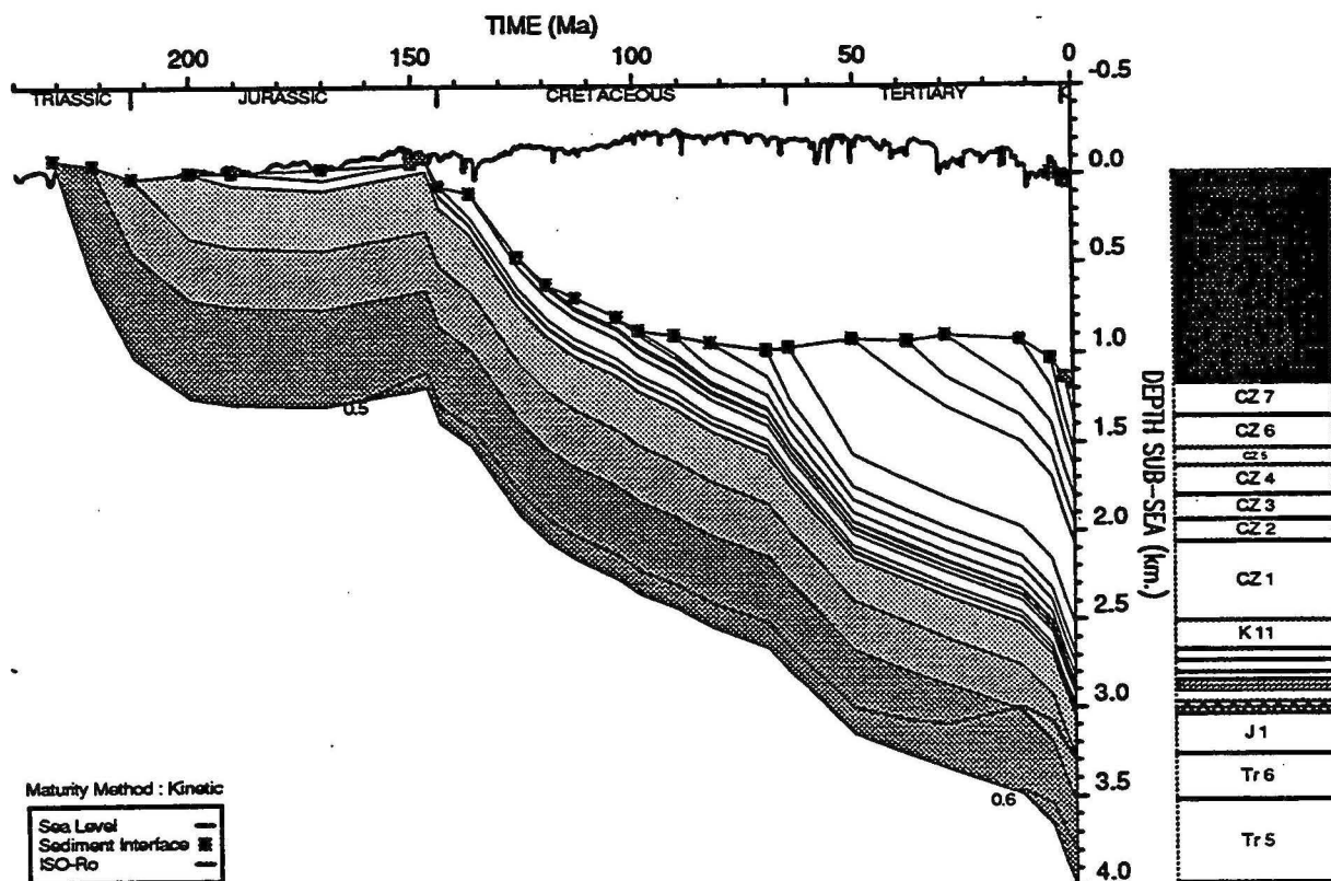
GEOHISTORY PLOT : Saturn 1
