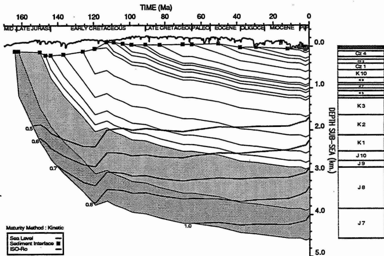
GEOHISTORY PLOT : Bambra 2
